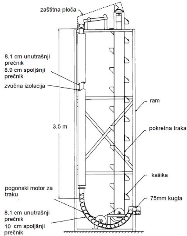
Slika 1 Uređaj za ispitivanje udarnog habanja kugli za mlevenje naizmeničnim sudarima kugla-kugla.
